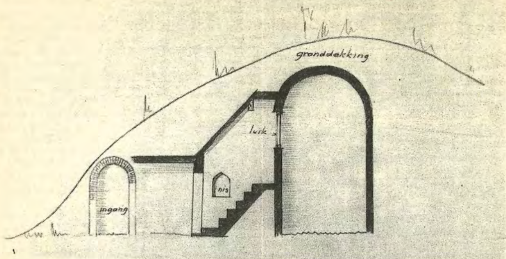
LENGTEDOORSNEDE IJSKELDER
