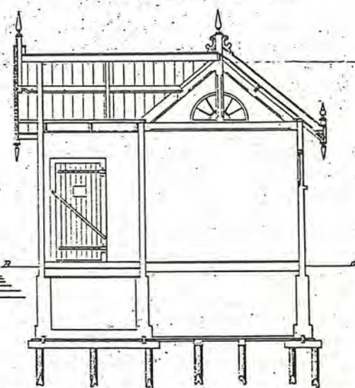
Leigte Doorsnede.
