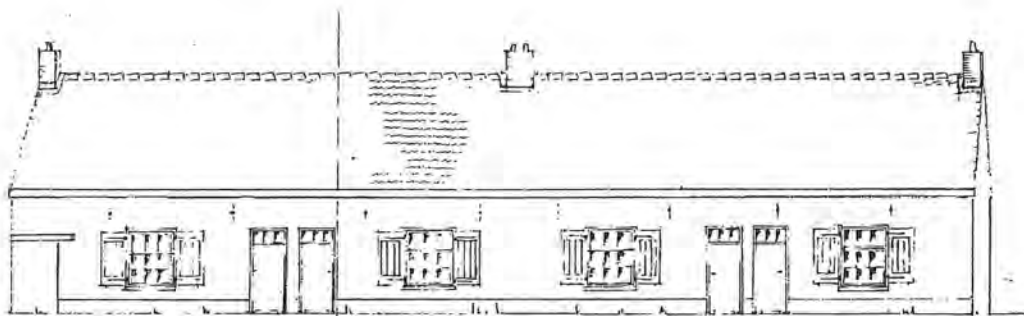
Reconstructie zuid(west)gevel Het Klooster omstreeks 1753.
