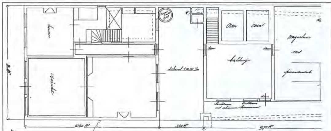
Afb.5: Bouwtekening uit 1904 van het huis en de bakkerij aan de Kerkweg. (Archief gem. Maarssen)
