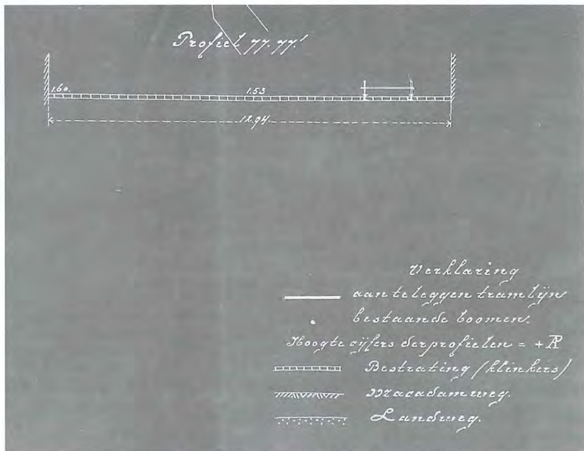
Afb. 2 Profiel van de Parkweg rond 1900, deels landweg, deels macadamweg. Afkomstig van de blauwdruk gemaakt voor de nooit aangelegde elektrische tramlijn Utrecht-Maarssen 1906. RHC Vecht en Venen, gemeente Maarssen, 1813-1938, inv. nr. 712
